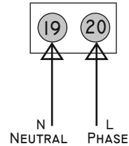
KLEMMENBRETT 4
